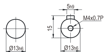
轴型式 S1
